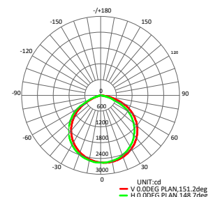
LF42- 49W/6704lm
