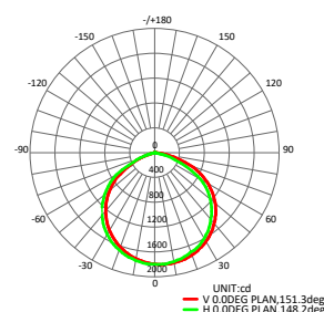
LF42- 31W/4924lm
